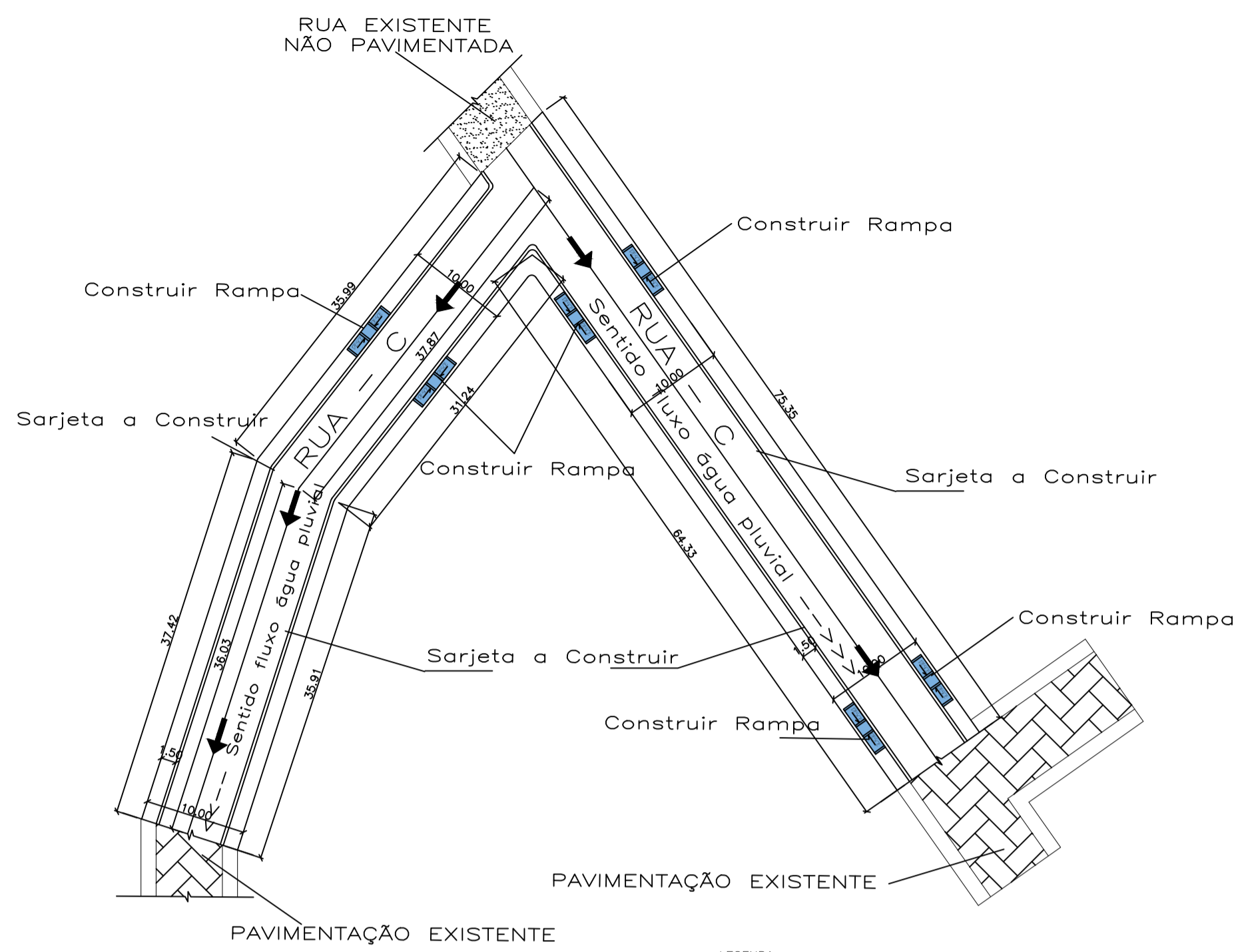
PLANTA DE DRENAGEM ESCALA: 1/500
