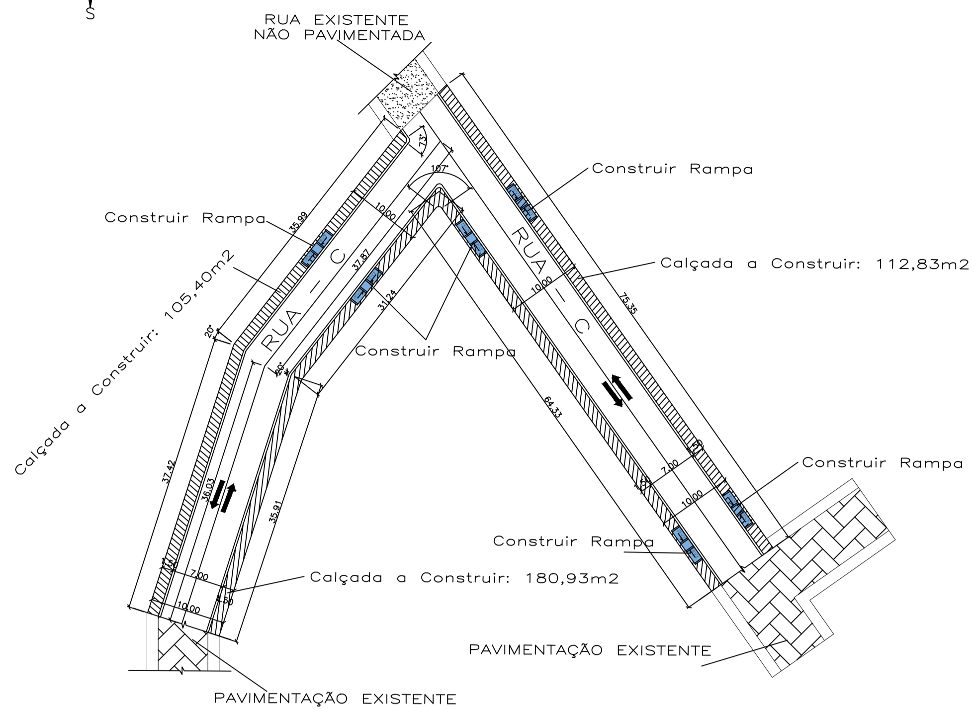
PLANTA DE CALÇADAS ESCALA: 1/500
