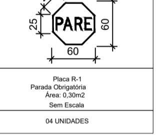
DET. SINALIZAÇÃO VERTICAL SEM ESCALA
