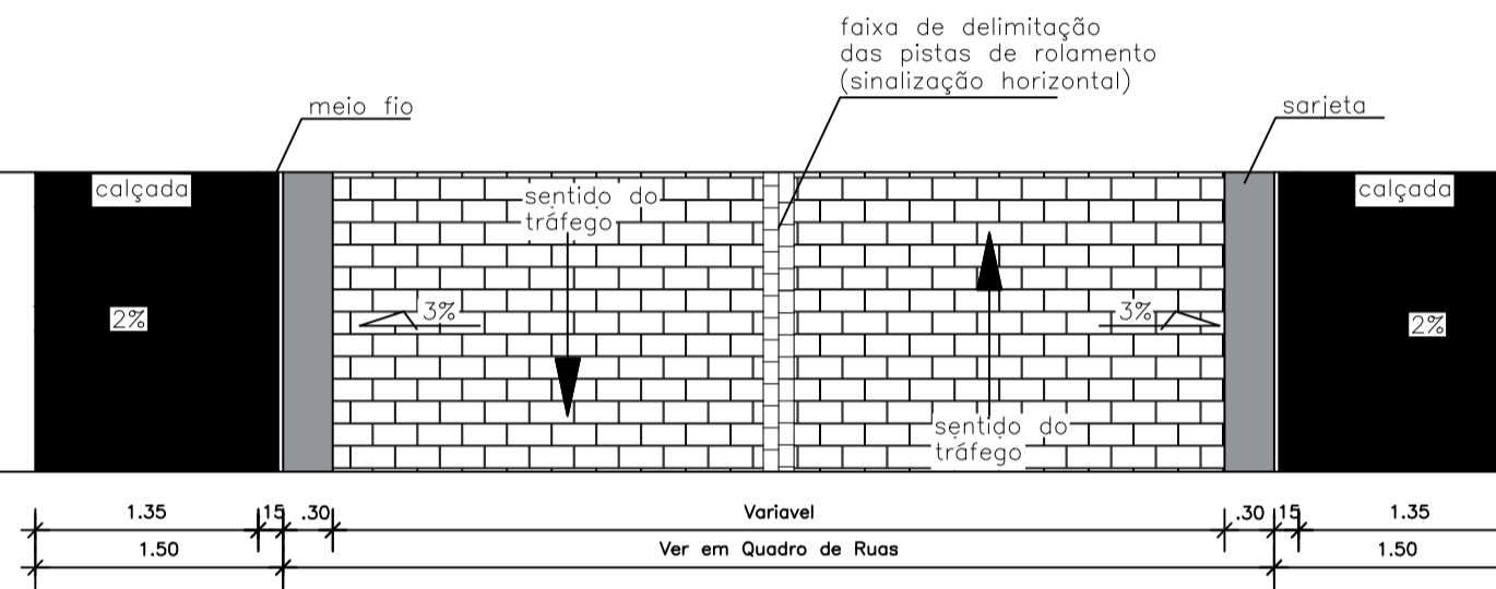
DET. PISTA ROLAMENTO ESCALA: 1/75
