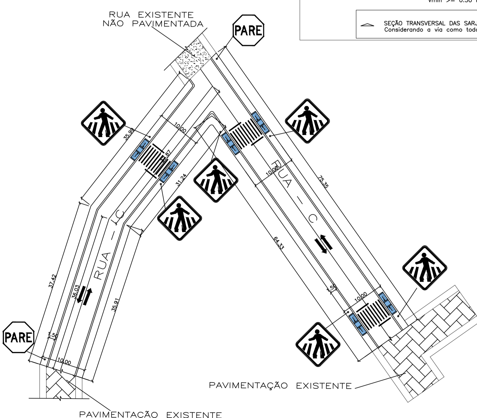
PLANTA DE SINALIZAÇÃO ESCALA: 1/500
