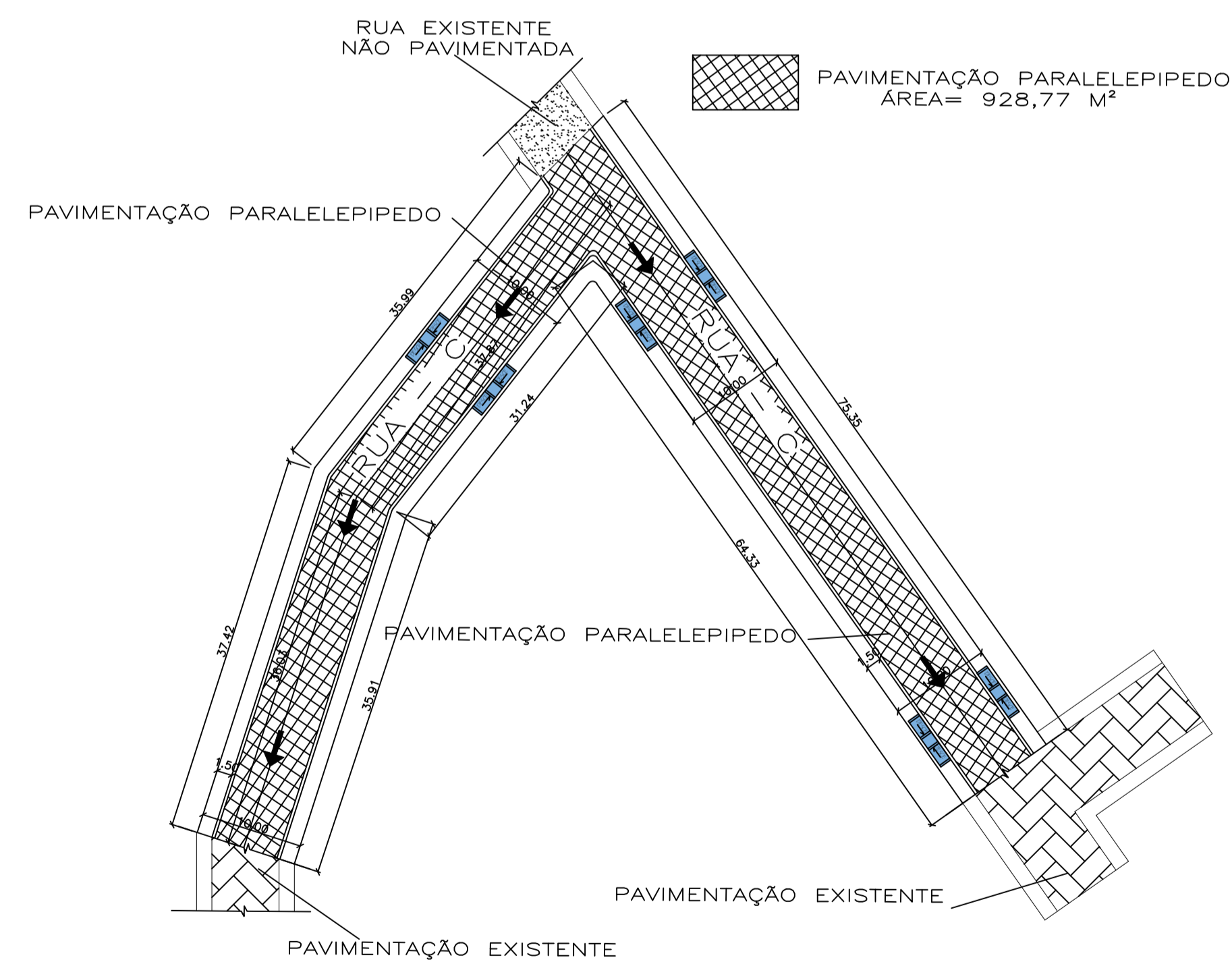
PLANTA DE PAVIMENTAÇÃO ESCALA: 1/500
