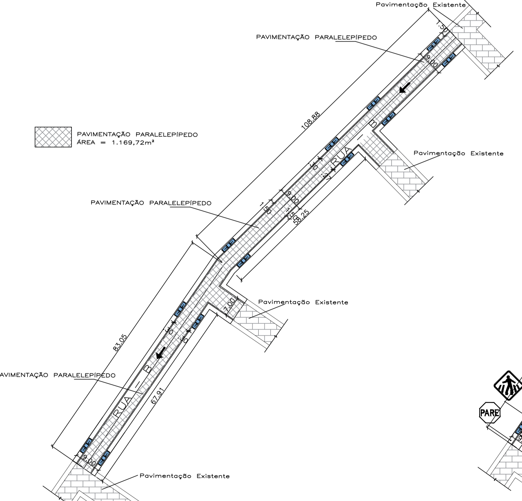
PLANTA DE PAVIMENTAÇÃO ESCALA: 1/750
