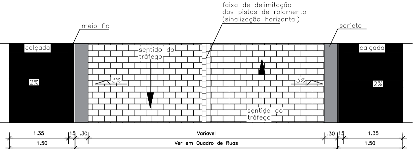
DET. PISTA ROLAMENTO ESCALA: 1/75
