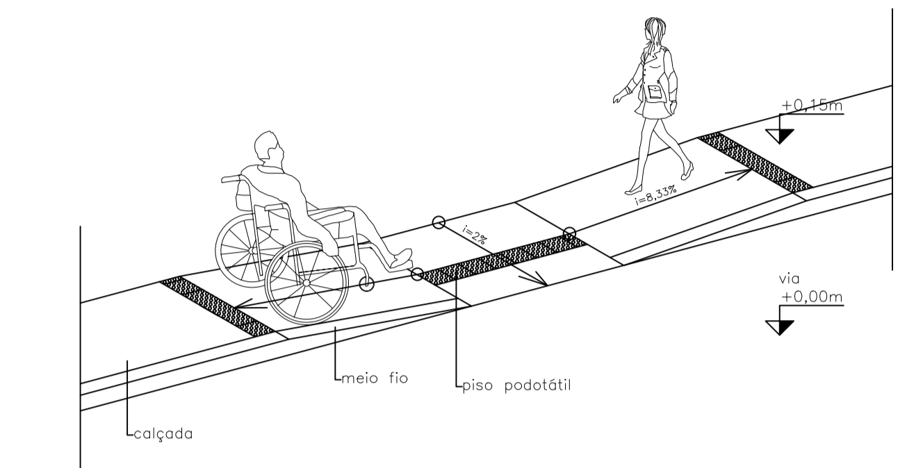
DET. RAMPA ESCALA: 1/75
