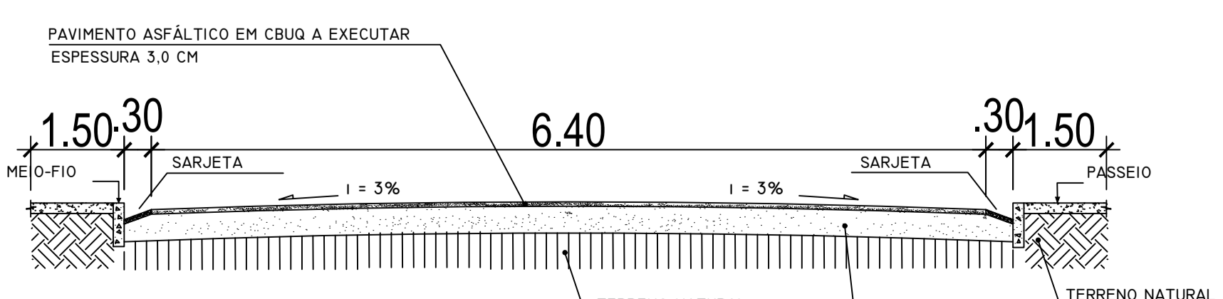
CORTE DE VIA ESCALA: 1/50
