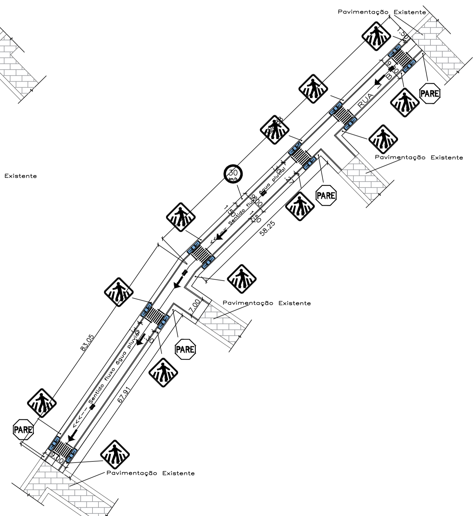
PLANTA DE SINALIZAÇÃO ESCALA: 1/750
