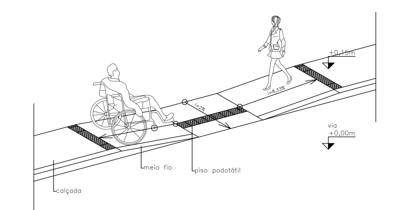
DET. RAMPA ESCALA: 1/75
