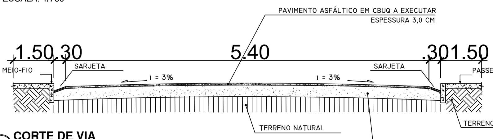
CORTE DE VIA ESCALA: 1/50
